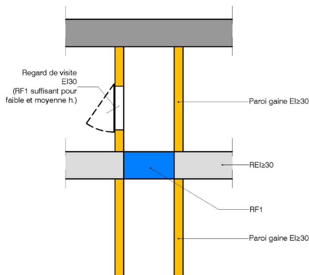
Gaine min. EI 30 avec séparation RF1 étanche à chaque niveau
