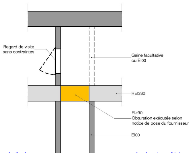
Traversées de plafonds réalisées comme une ouverture et trémie de câbles et de tuyaux
