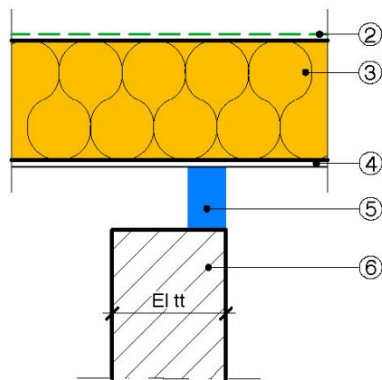
Coupe A-A
