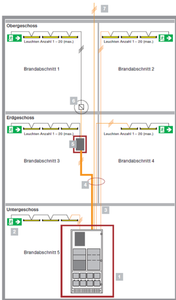
Schéma du câblage dans les différents compartiments coupe-feu
