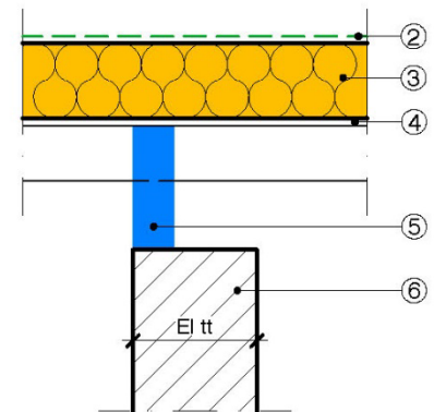
Coupe B-B
